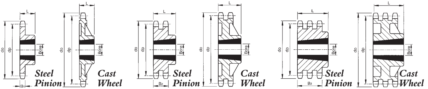
Simplex Sprockets Chain No. 06B-1
