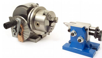
Przyrząd podziałowy z konikiem
