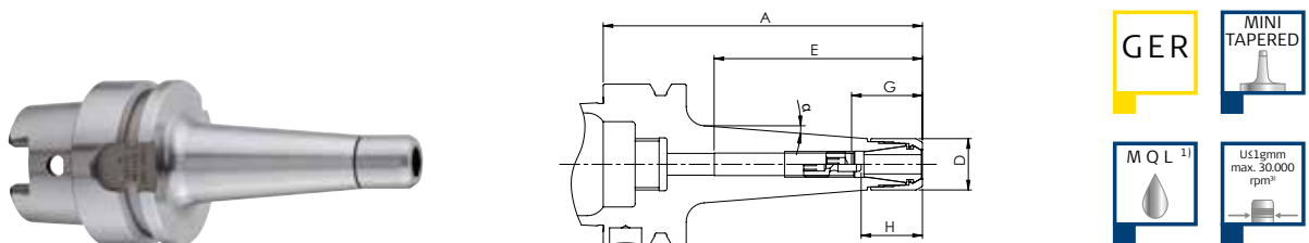
CENTRO|P – Tapered Version for HPCM Mini Clamping Nuts
