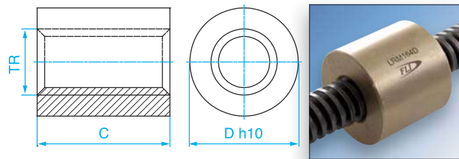
Ecrou cylindrique en bronze Nuance CC493K(CuSn7ZnPb) ROHS sur consultation
