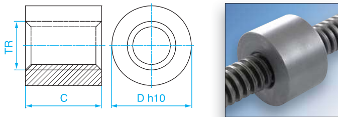
Ecrou cylindrique en acier Nuance 11SMnPb37
