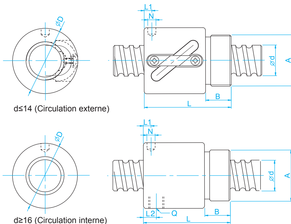
Classe de précision C7 / Grade C7
