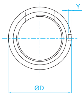
Classe de précision C7 / Grade C7
