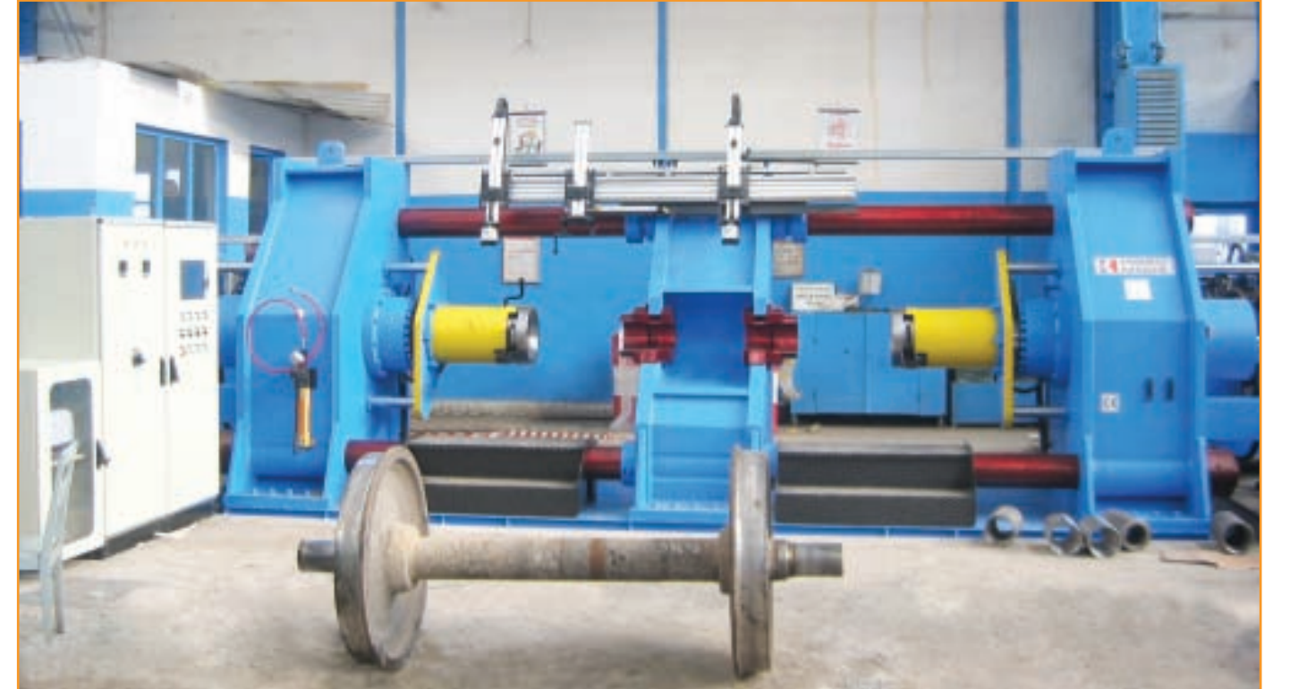
Demir Yolları için Dingil Çakma Presi Spindle Assmbling Press for Railway Association
