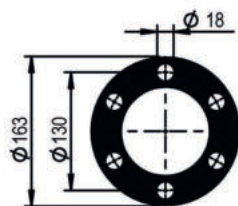
Rundflansch // round flange
