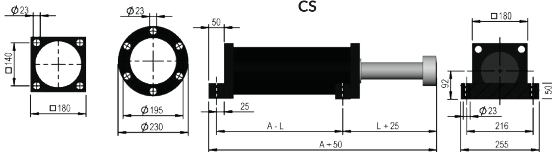
Quadratflansch // square flange
