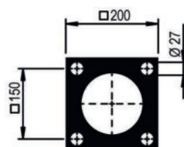
Quadratflansch // square flange
