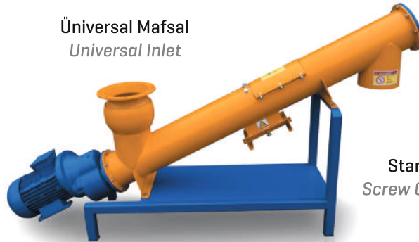
Çimento Helezonu Cement Screw Conveyor
