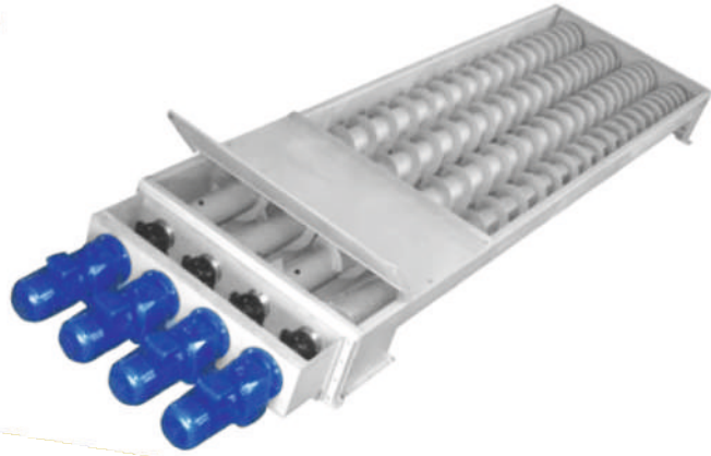
Treme Havuzu Kademeli Boşaltma Helezonu Treme Pondage Stepping Discharge Screw Conveyor
