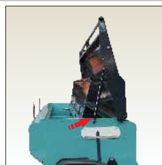
Tramoggia con martinetto idraulico Hopper with hydraulic jack Trémie avec vérin hydraulique Tolva con gato hidráulico
