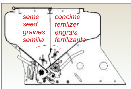
Pannello mobile per tramoggia seme/concime - Detachable seed/fertilizer hopper panel Panneaux mobiles pour trémie graines/engrais - Consola móvil para tolva semilla/fertilizante
