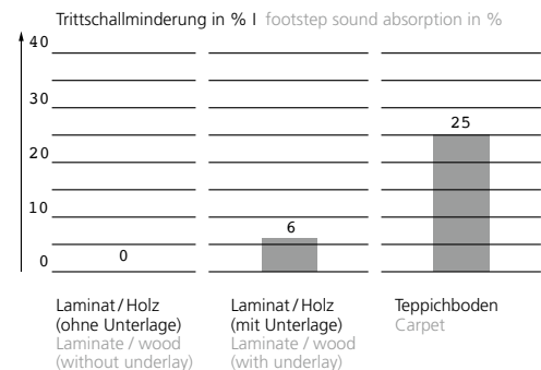
Grafik: Minderung des Trittschalls durch die Verwendung von Teppichboden im Vergleich zu Laminat und Holzboden um bis zu 40%. (Quelle: TFI, Aachen) Graphics: Reduction of footstep sound by using carpets compared with laminates and granolithic floors by up to 40%. (Source: TFI, Aachen)
