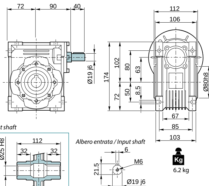
VI 063 P ...
