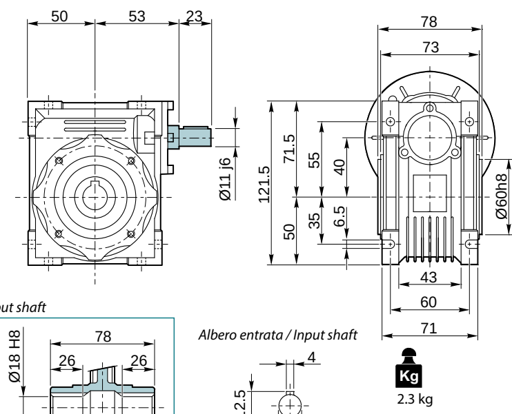
VI 040 P ...
