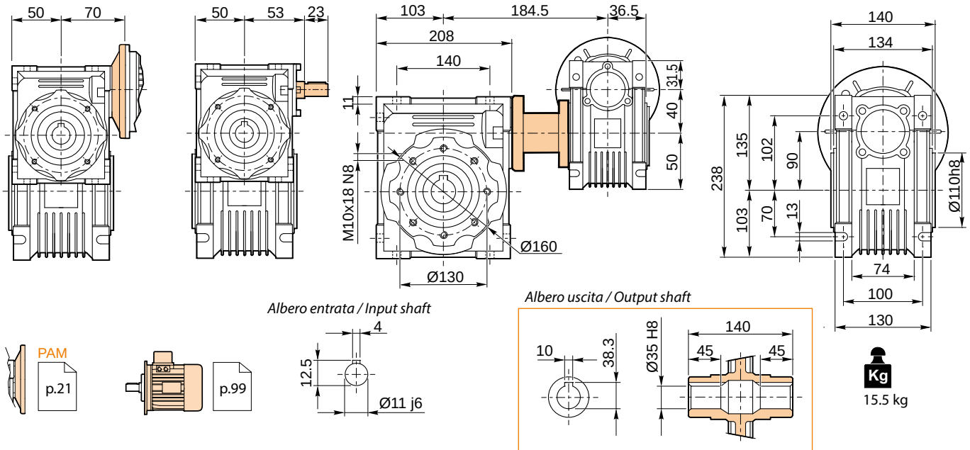
VC 040 / 090 F...
