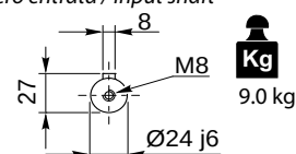
Albero entrata / Input shaft
