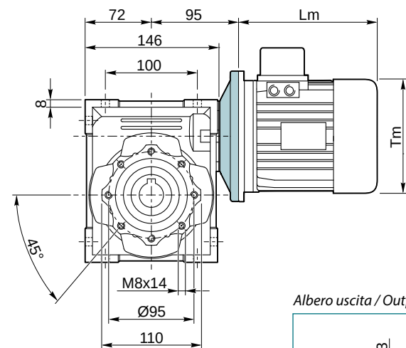
VP 063 P ...
