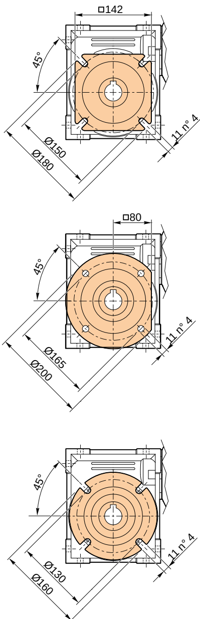
VC 030 / 063 F...
