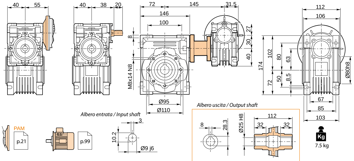
VC 030 / 063 F...
