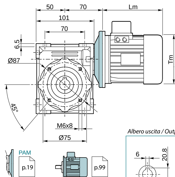
VP 040 P ...
