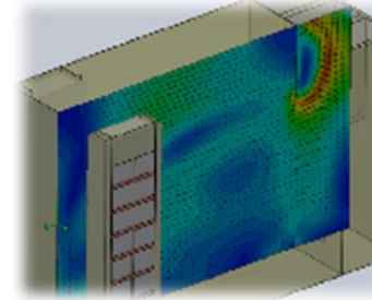
Akış ve Isı Transfer Analizi
