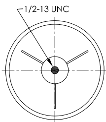
ALU PISTON
