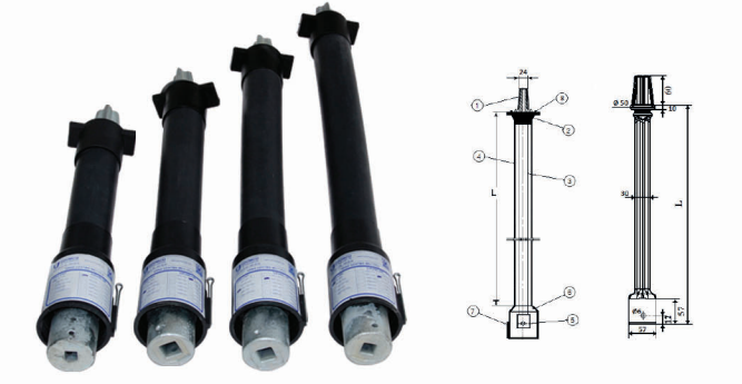
VANA UZATMA MİLİ (Tij)
