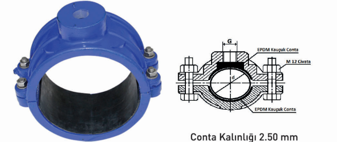
PRİZ KOLYE (Sfero Döküm)
