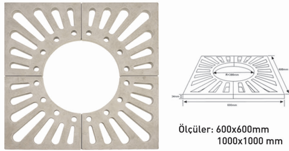
AĞAÇ ALTI MAZGALI
