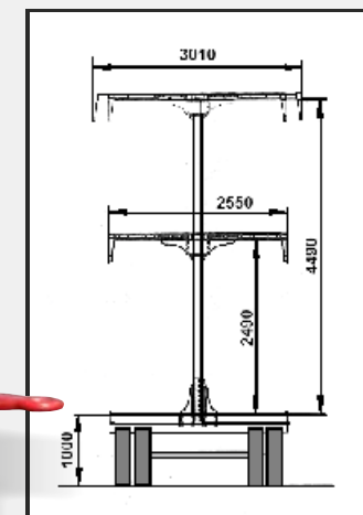
allargamenti laterali compressione rotoballe
